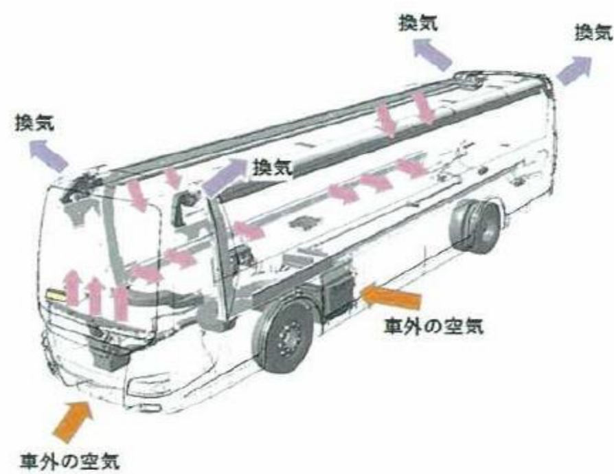
大型観光バス・床下A/Cタイプ
